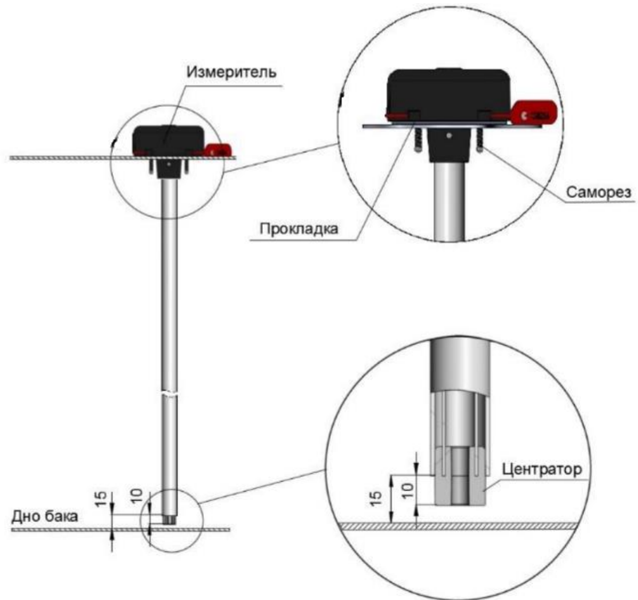
Рис. 12.3. Монтаж измерителя на бак
